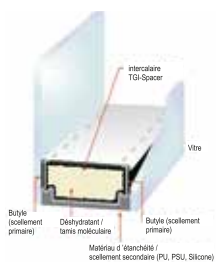
Coupe de l'intercalaire Warm Edge
